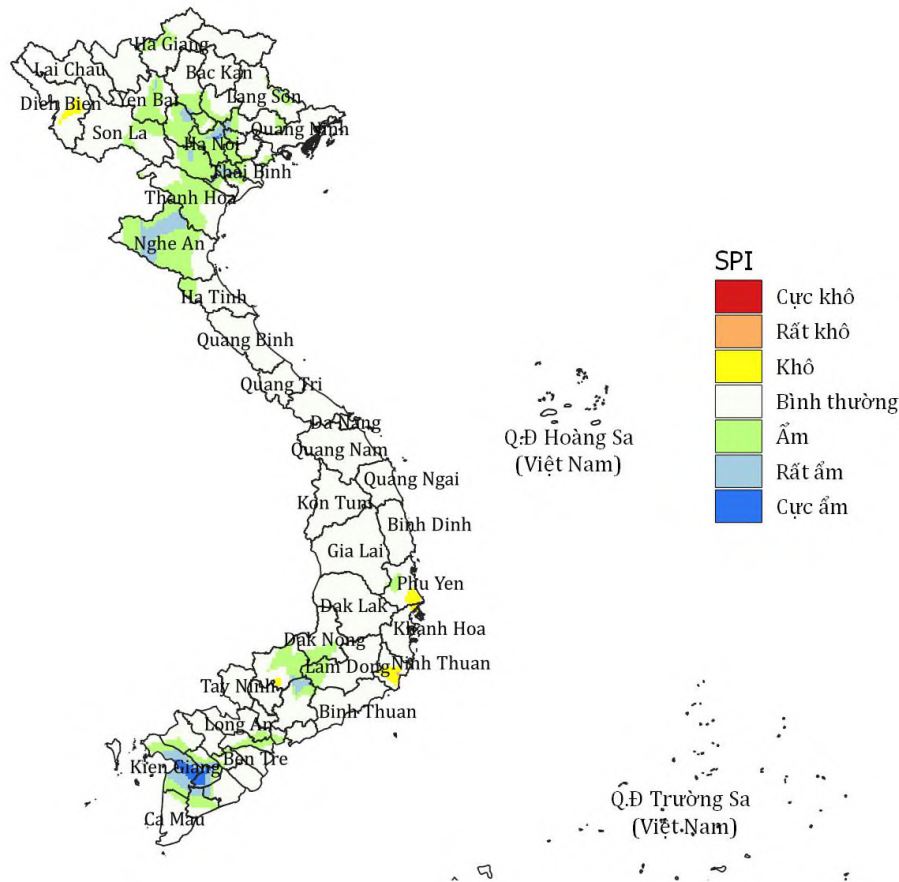
Hình 2: Chỉ số SPI biểu thị điều kiện khô hạn hay ẩm ướt từ 01-29/9/2023. Điều kiện khô hạn (gam màu vàng – đỏ), điều kiện ẩm ướt (gam màu xanh).
