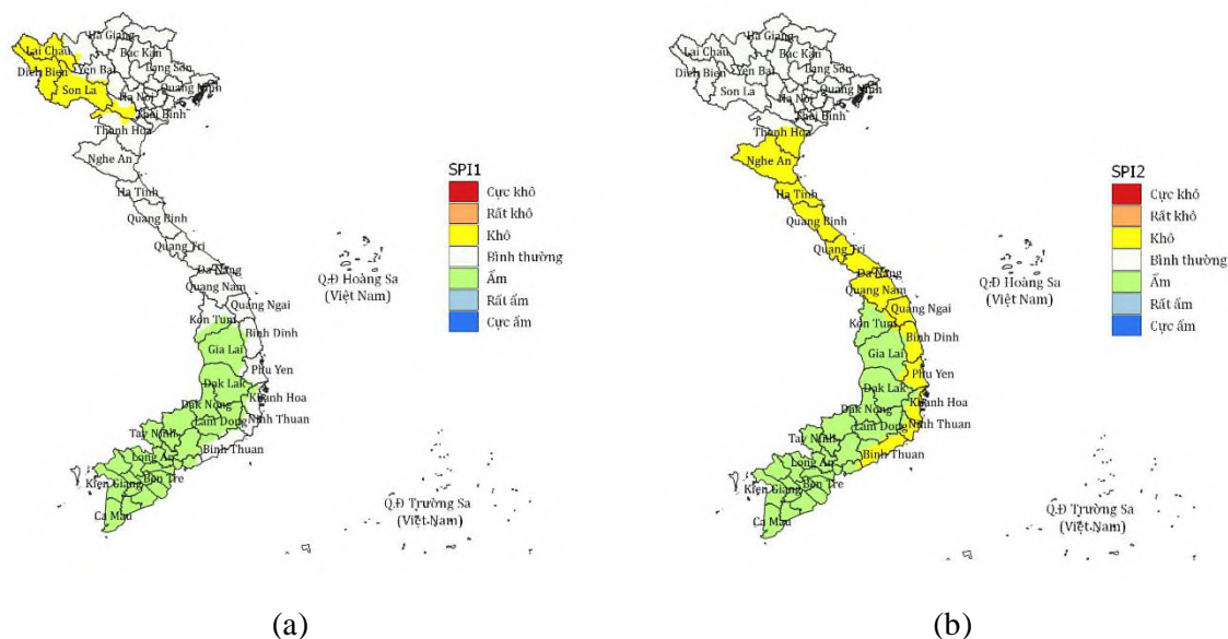
Hình 3: Chỉ số SPI biểu thị điều kiện khô hạn hay ẩm ướt từ ngày 01-15/10(a); và từ ngày 16-31/10/2023(b).
