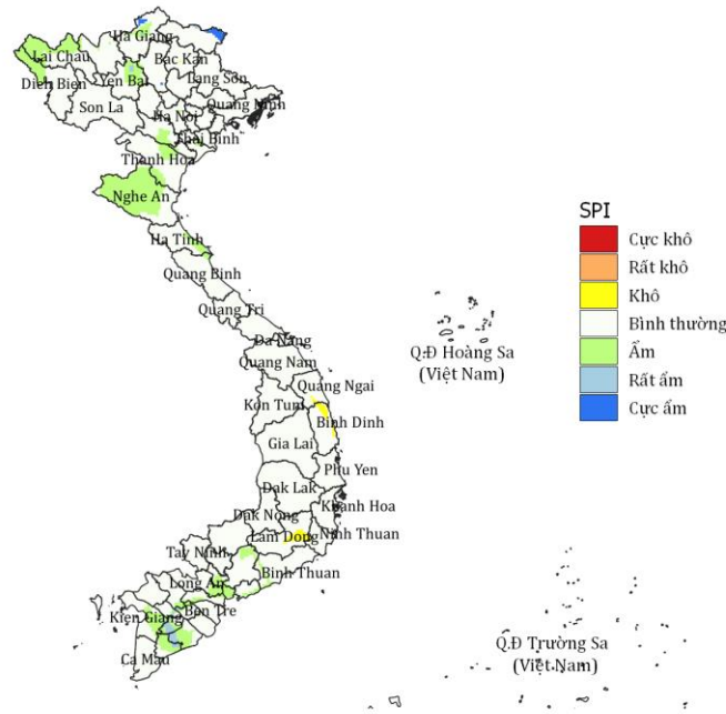
Hình 2: Chỉ số SPI biểu thị điều kiện khô hạn hay ẩm ướt từ 15/9-15/10/2023. Điều kiện khô hạn (gam màu vàng – đỏ), điều kiện ẩm ướt (gam màu xanh).
