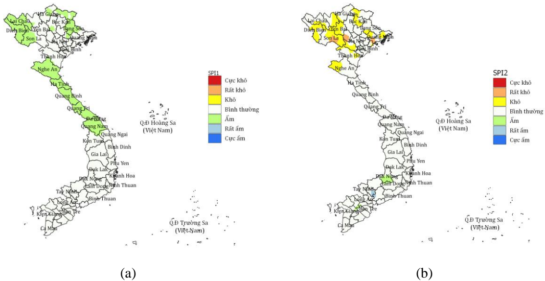
Hình 3: Chỉ số SPI biểu thị điều kiện khô hạn hay ẩm ướt từ ngày 16-31/10(a); và từ ngày 01-15/11/2023(b).
