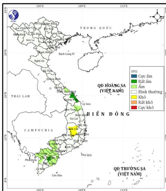
Hình 3: Chỉ số SPI đánh giá tình trạng ẩm ướt và khô hạn giai đoạn từ 14-31/5/2022. Gam màu xanh là điều kiện ẩm, gam màu vàng – đỏ là điều kiện khô hạn
