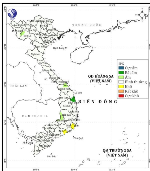
Hình 4: Chỉ số SPI đánh giá tình trạng ẩm ướt và khô hạn giai đoạn từ 01-15/4/2022. Gam màu xanh là điều kiện ẩm, gam màu vàng – đỏ là điều kiện khô hạn
