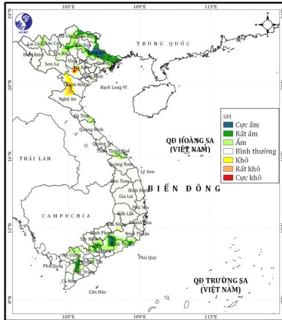
Hình 2: Chỉ số SPI biểu thị điều kiện khô hạn hay ẩm ướt từ ngày 15/4-13/5/2022. Điều kiện khô hạn (gam màu vàng – đỏ), điều kiện ẩm ướt (gam màu xanh)
