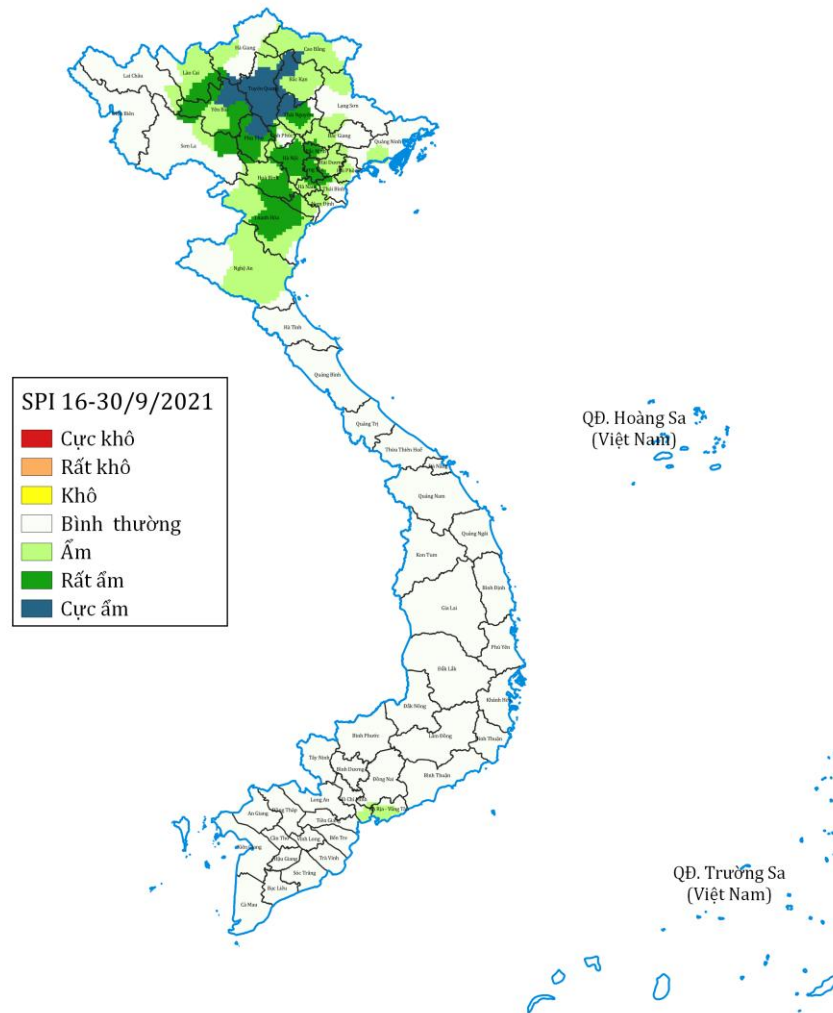
Hình 3: Chỉ số SPI đánh giá tình trạng ẩm ướt và khô hạn giai đoạn từ 16-30/9/2021. Gam màu xanh là điều kiện ẩm, gam màu vàng – đỏ là điều kiện khô hạn
