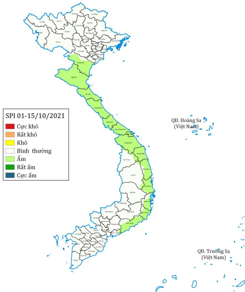
Hình 4: Chỉ số SPI đánh giá tình trạng ẩm ướt và khô hạn giai đoạn từ 01-15/10/2021. Gam màu xanh là điều kiện ẩm, gam màu vàng – đỏ là điều kiện khô hạn
