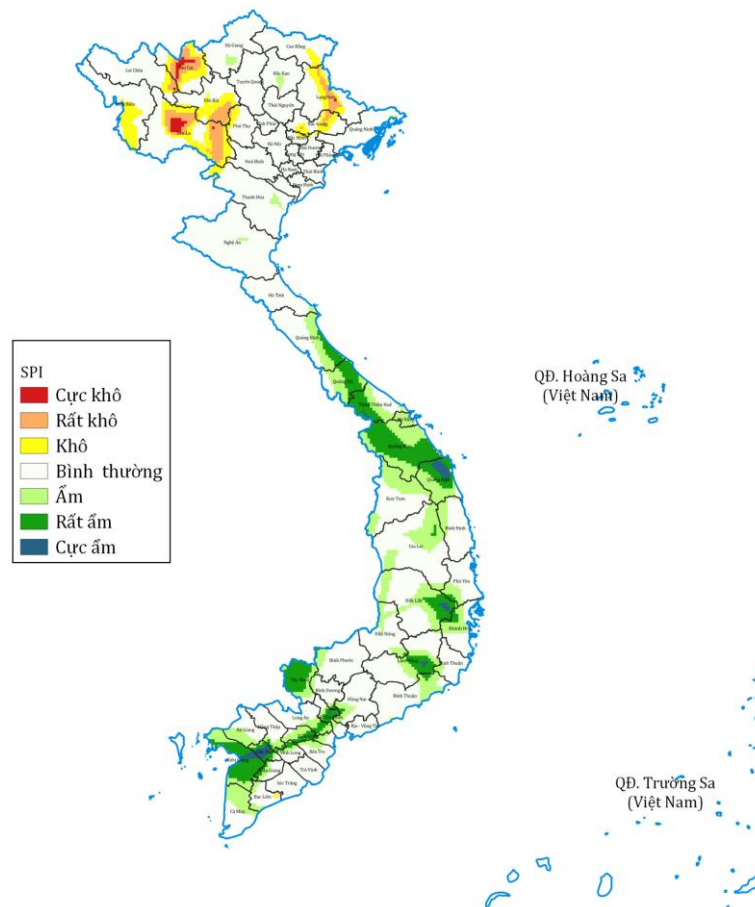
Hình 2: Chỉ số SPI biểu thị điều kiện khô hạn hay ẩm ướt trong thời kỳ 15/8-15/9/2021. Điều kiện khô hạn (gam màu vàng – đỏ), điều kiện ẩm ướt (gam màu xanh)
