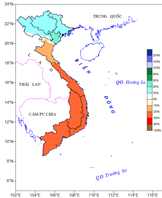
Tỷ chuẩn lượng mưa dự báo từ ngày 21/6-20/7/2021
