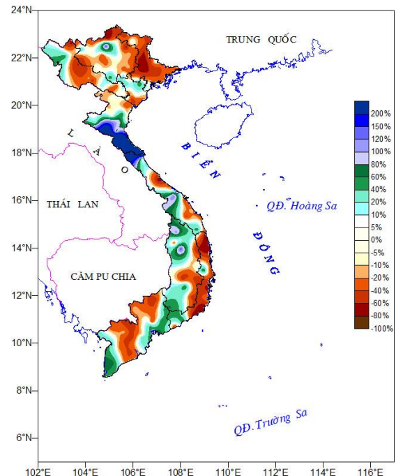
Tỷ chuẩn lượng mưa từ ngày 21/5-20/6/2021
