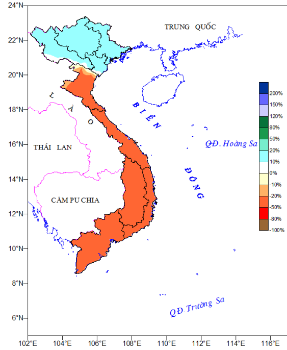
Tỷ chuẩn lượng mưa dự báo từ ngày 01-10/7/2021
