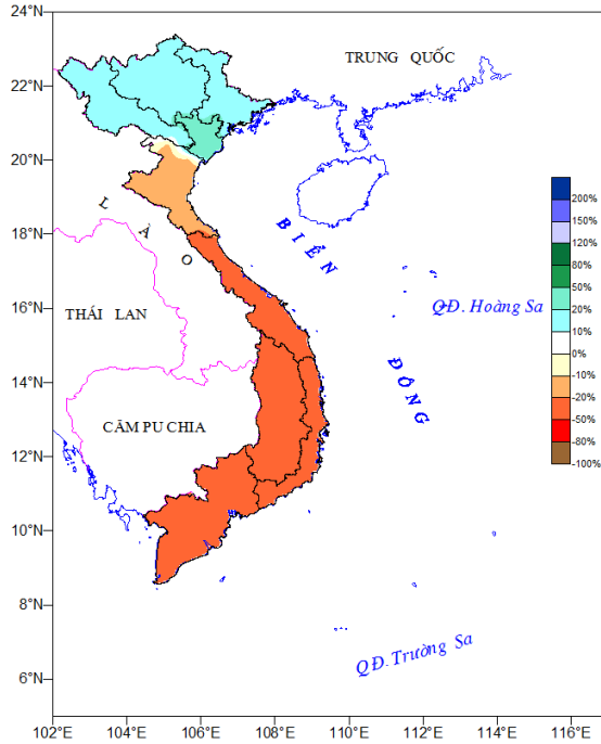
Tỷ chuẩn lượng mưa dự báo từ ngày 21-30/6/2021
